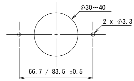
取付穴加工図 (参考)
