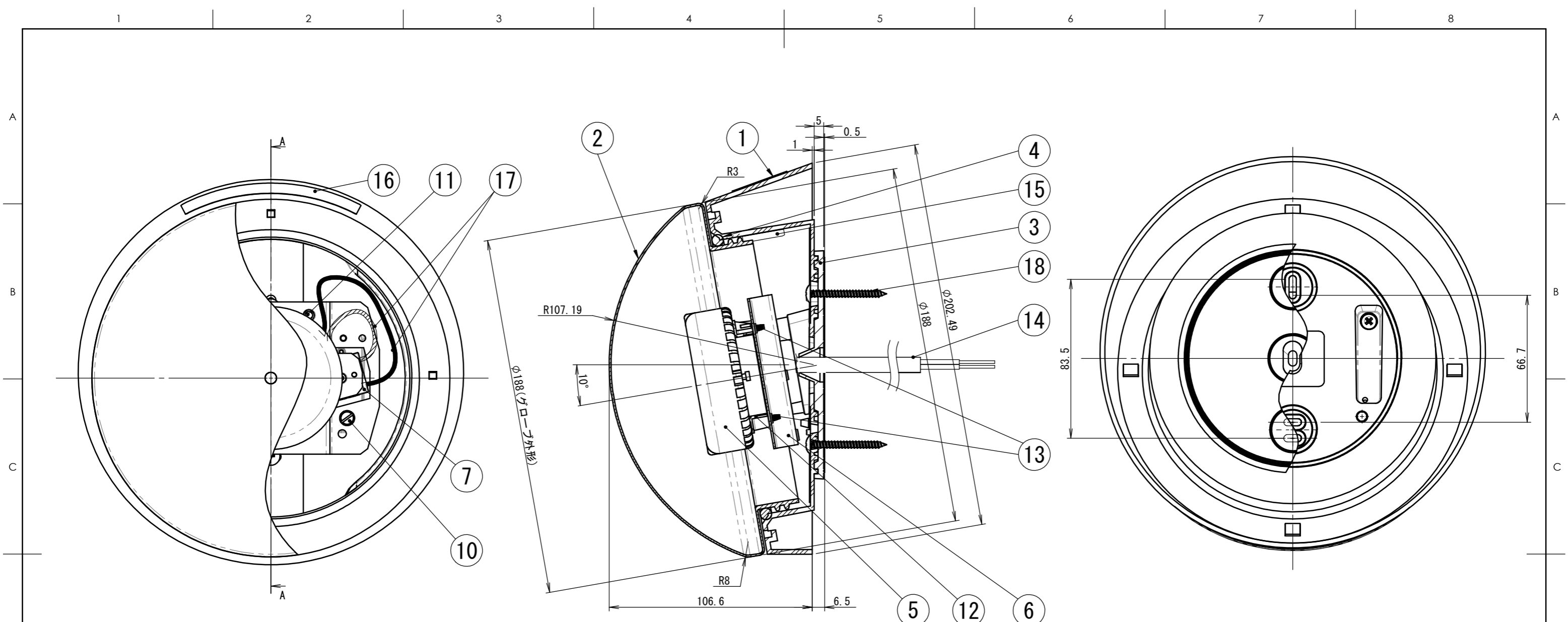
断面図 A-A
