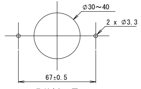
取付穴加工図
