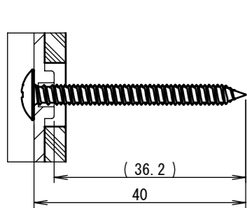
断面図 A-A スケール 1 : 1
