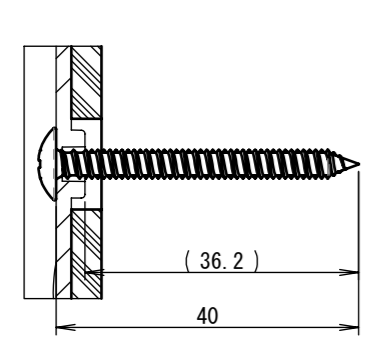
断面図 A-A スケール 1 : 1
