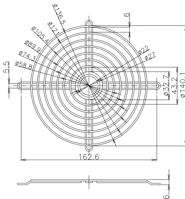
■150φ用 RG150-7T
