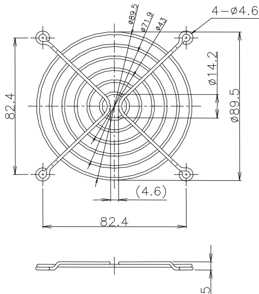
■92角用 RG92-6
