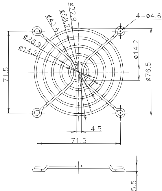
■80角用 RG80-5
