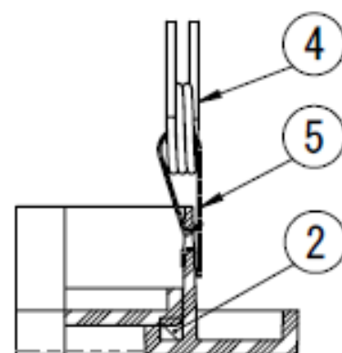
詳細図 A 尺度 1 : 1
